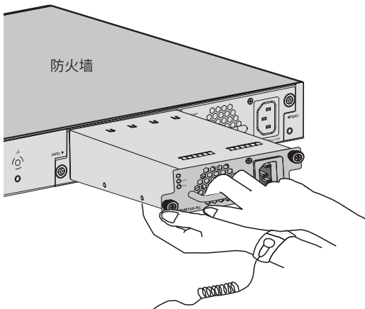
图3-7 安装电源模块示意图
