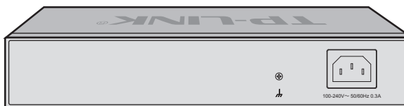
图1-4 TL-FW5600后面板示意图
