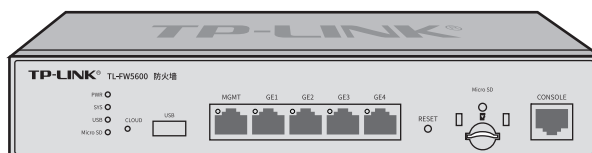
图1-2 TL-FW5600前面板示意图
